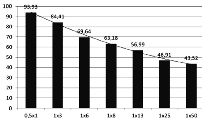
Рис. 2. Диаграмма изменения расчетного практического выхода концентрата коксующегося угля пласта N16 для различных машинных классов крупности при исходной пластовой зольности 22,4 %
