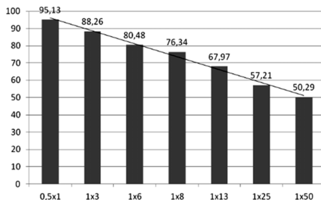
Рис. 3. Диаграмма изменения расчетного практического выхода концентрата коксующегося угля пласта У4 для различных машинных классов крупности при исходной пластовой зольности 23,97 %
