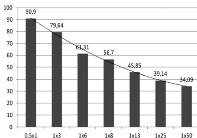
Рис. 1. Диаграмма изменения расчетного практического выхода концентрата коксующегося угля пласта N15 для различных машинных классов крупности при исходной пластовой зольности 35,0 %
