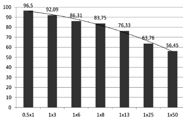
Рис. 4. Диаграмма зависимости расчетного практического выхода концентрата коксующегося угля пласта У5 для различных машинных классов крупности при исходной пластовой зольности 26,73 %
